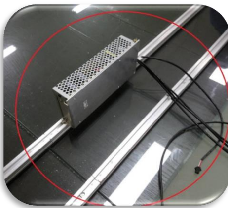
圖五、放 6 個螺帽的橫桿其中二個螺帽固定電源(自行調整電源固定位置以避開燈箱相互干涉到)
