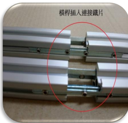
圖二、橫桿插入連接鐵片, 4支約1米長橫桿接成2支
