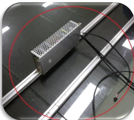
圖八、放6個螺帽的橫桿其中二個螺帽固定電源(自行調整電源固定位置以避開燈箱相互干涉到)
